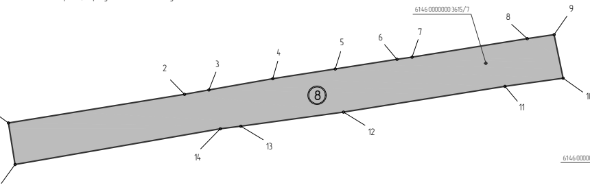
Чертеж межевания территории с обозначением границ образуемого земельного участка №8 (М 1:1000)
